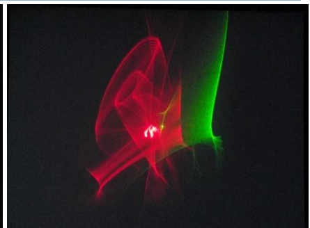
おどる光の干渉模様
