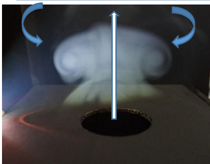
空気砲が作る煙のうず
