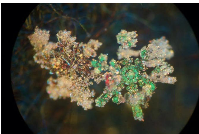
雲粒つき
