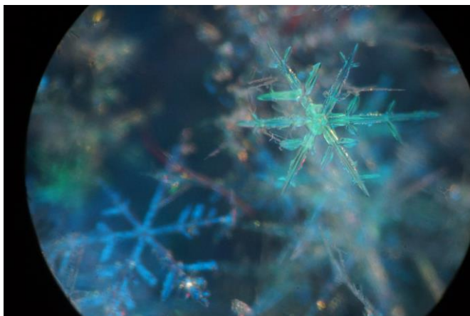
樹枝六花
