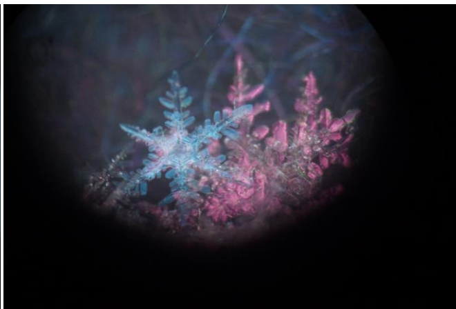
羊歯六花
