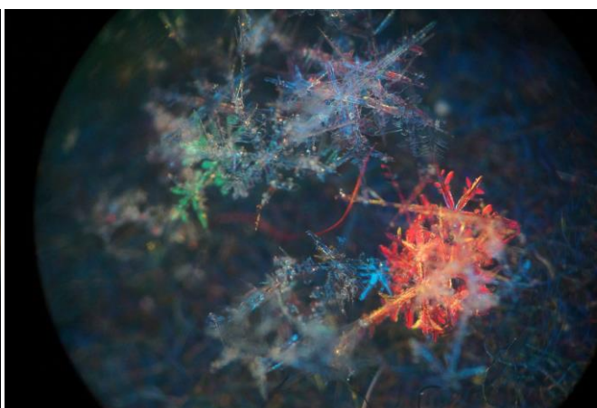
ぼたん雪
