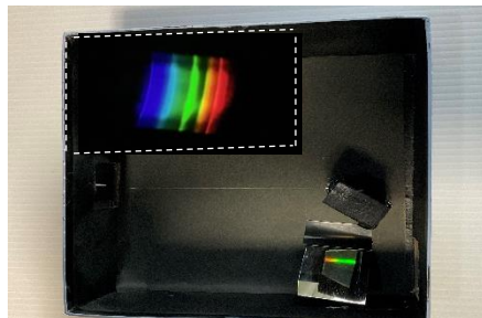
手作り CD 分光器で光のスペクトル
